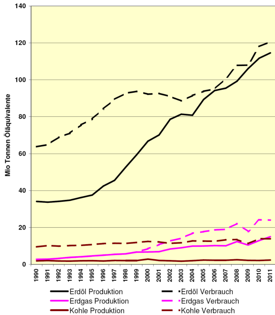
Brasilien Erdöl, Erdgas, Kohle Produktion und Verbrauch 1990 - 2011
