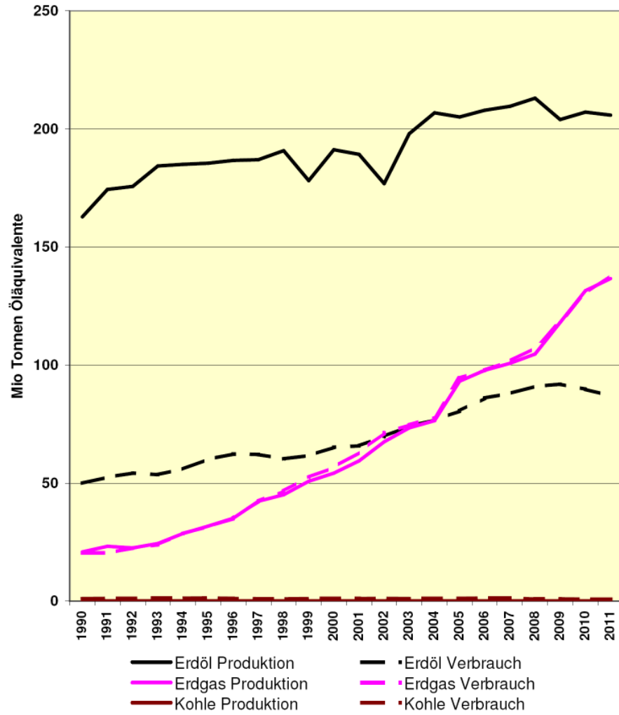
Iran Erdöl, Erdgas, Kohle Produktion und Verbrauch 1990 - 2011
