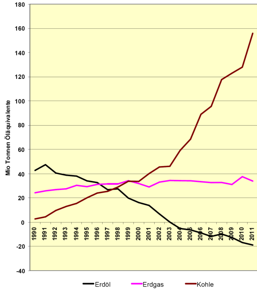
Indonesien Erdöl, Erdgas, Kohle Bilanz Produktion - Verbrauch 1990 - 2011
