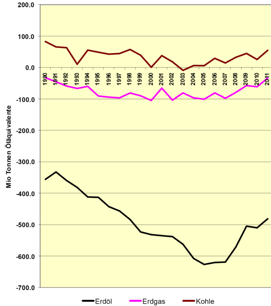
USA: Erdöl, Erdgas, Kohle Bilanz Produktion - Verbrauch 1990 - 2011
