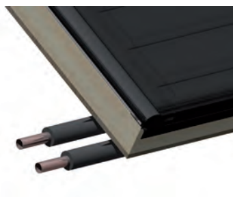
Anschlüsse in Lattenhöhe: Leitungen können unter den Dachziegeln verlegt werden (nur bei VarioSol E).
