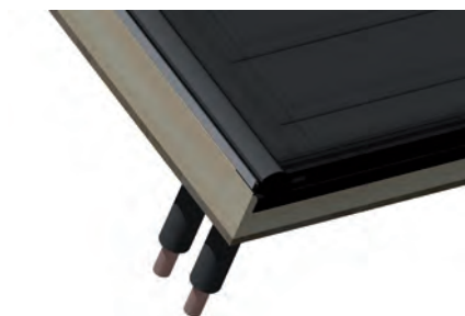
Anschlüsse durch die Rückwand: Anbindung vom Dachboden aus.
