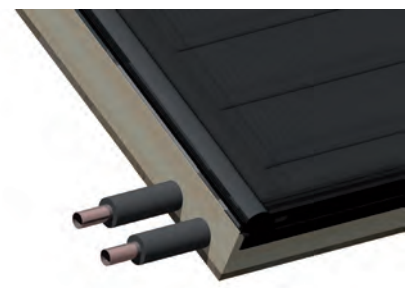
Anschlüsse durch den Kollektorrahmen: z.B. bei Fassadeneinbau (bei Indachmontage mit Eindeckrahmen nicht möglich).
