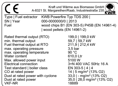
Muster eines Typenschilds
