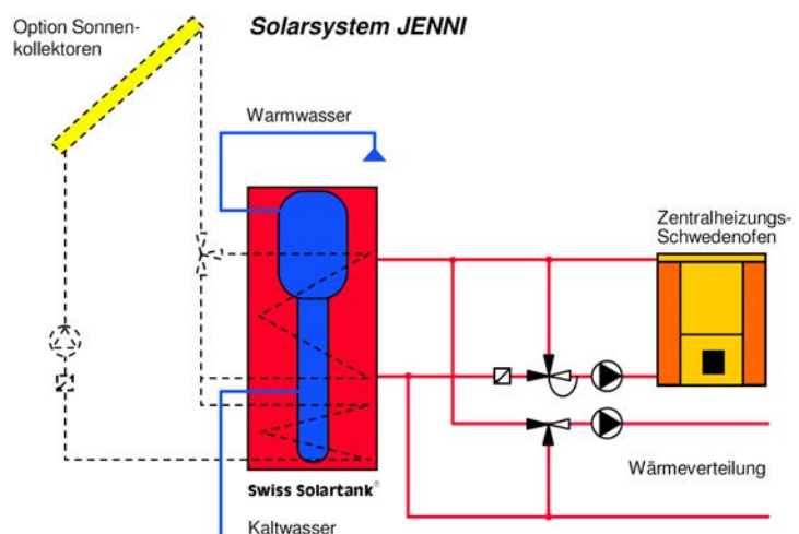
Beispiel Pinzipschema mit Sonnenkollektoren
