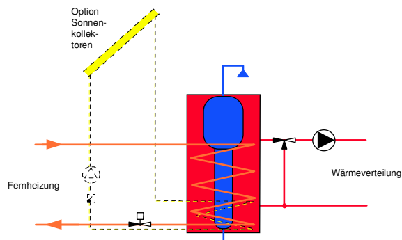
Fernheizungs-Hausstation mit Swiss Solartank ® , Wassererwärmer und Wärmetauscher integriert
