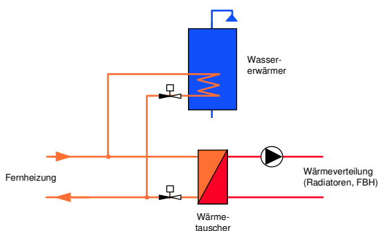
Konventionelle Anlage
