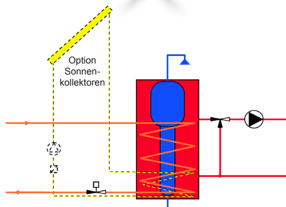
Nah-/Fernwärme-Hausstation System Jenni Wasserewärmer und Wärmetauscher integriert (Schema 1)
